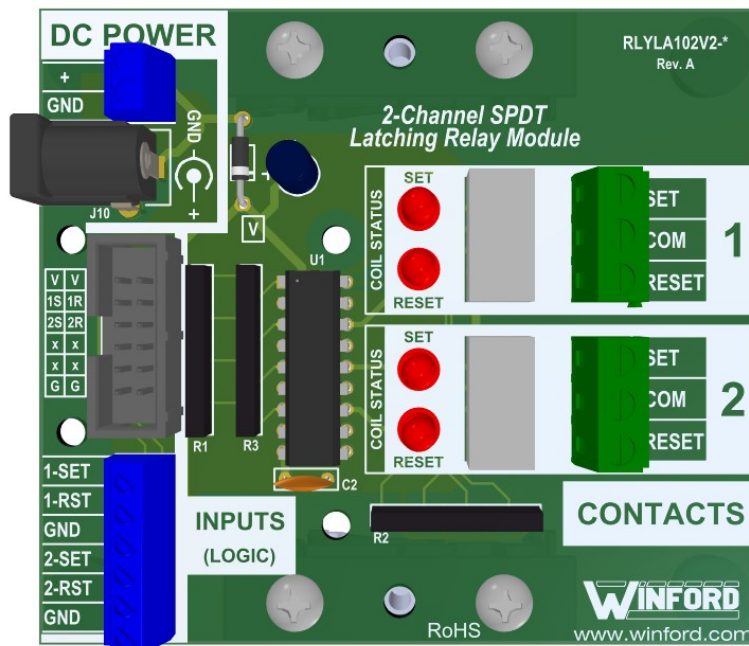
DIN Mounting Option Shown
