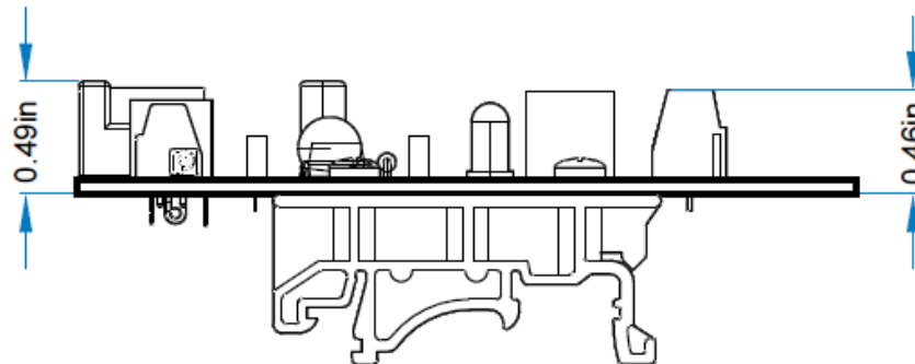
DIN Mounting Option Shown
