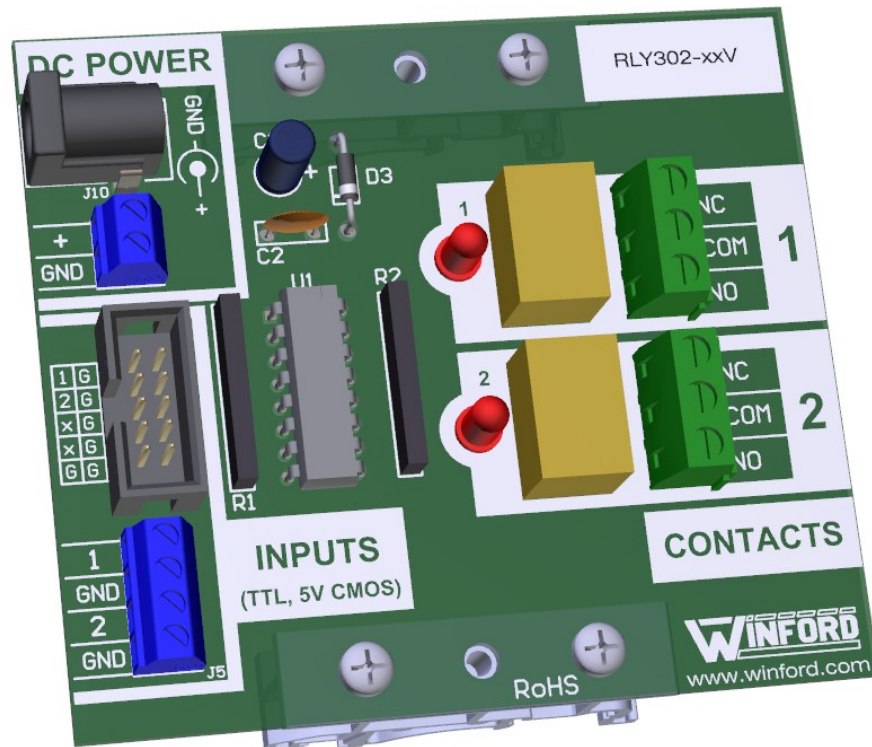
DIN Mounting Option Shown
