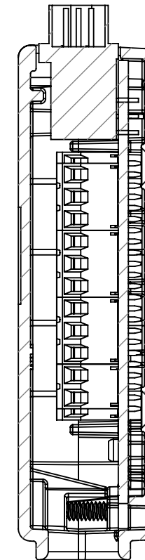
SECTION A-A
