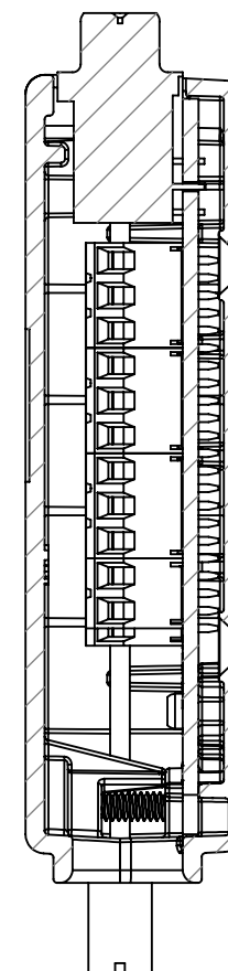
SECTION A-A
