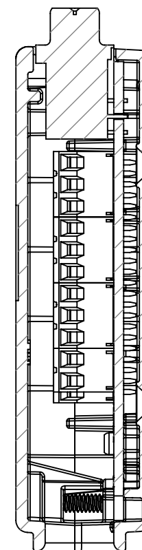
SECTION A-A
